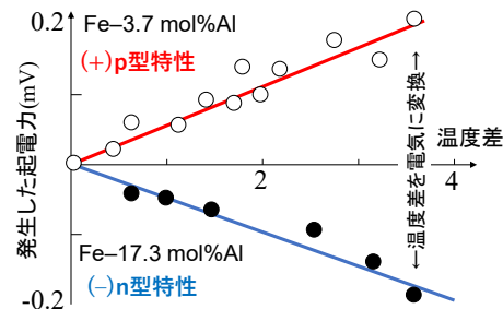
図. Fe-Al電析物の熱電効果
