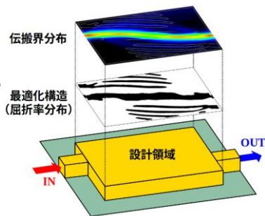
光回路の導波路構造最適化
