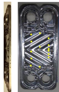
金属3Dプリンタによる 熱交換器プレート作成
