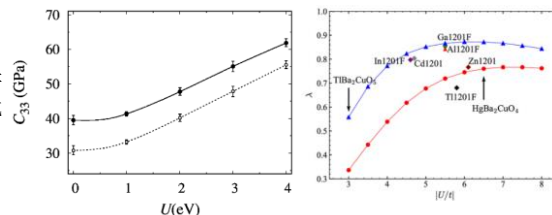
黒鉛の強相関パラメータ( U )と弾性定数[1]. U \sim 2.1 [eV]で実測に近い数値を与える。
