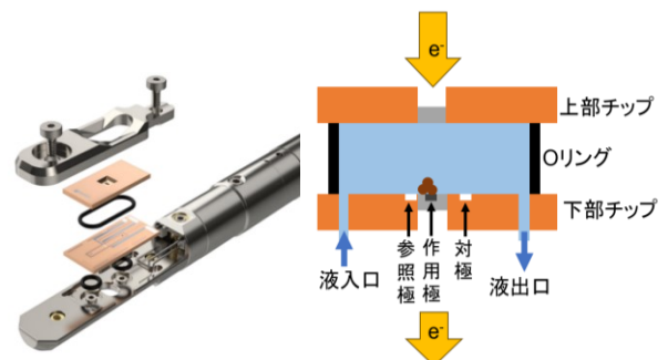
図 2 液中オペランド TEM 観察用試料ホルダーの構成と液体セルの模式図
