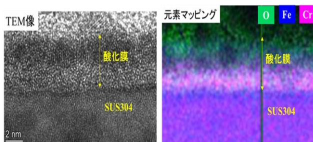
図 1 電解研磨した SUS304 ステンレス鋼の断面 TEM 像とその元素マッピング像
